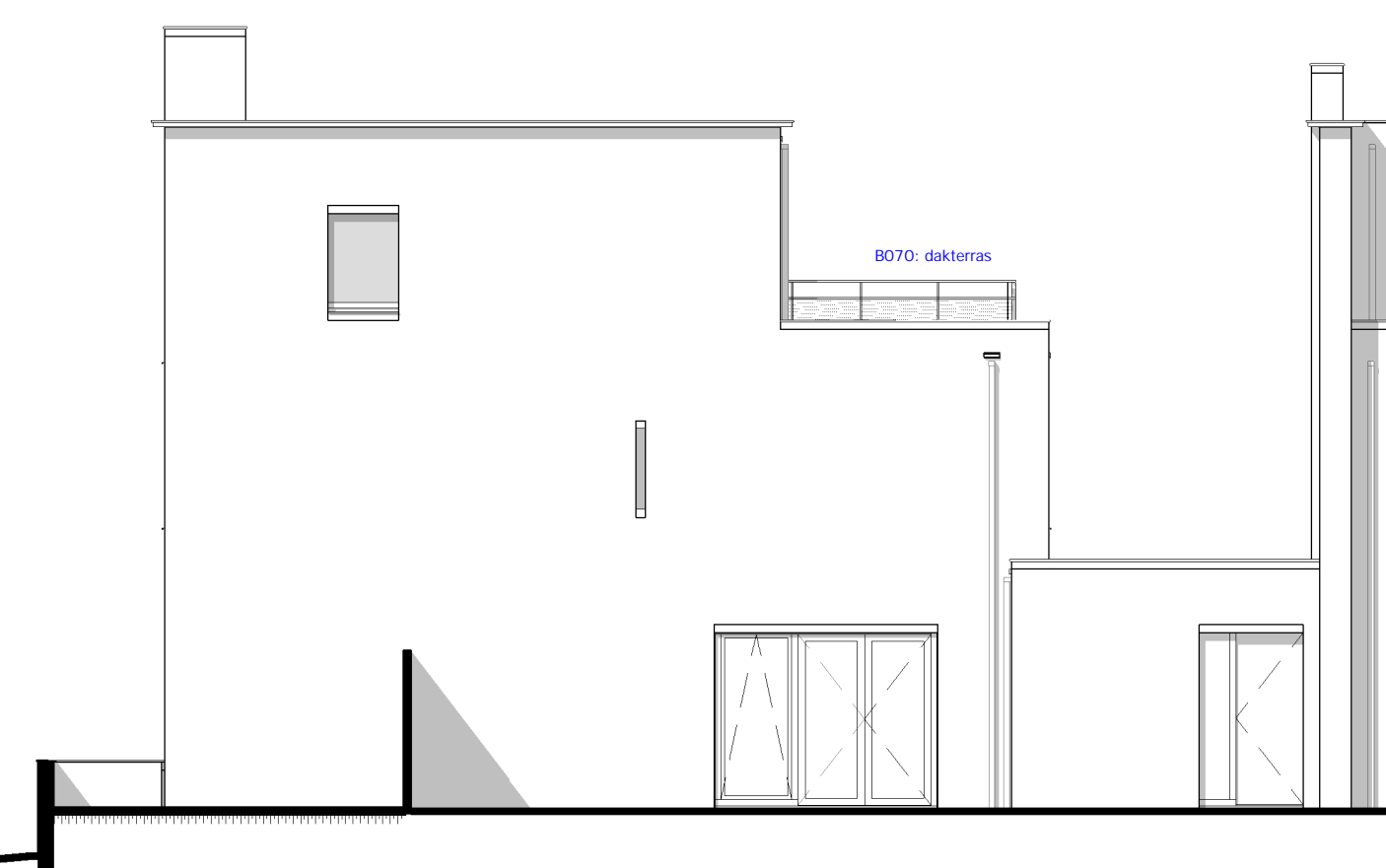
ENTREEGEVEL
