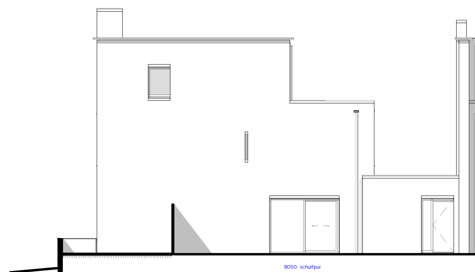
ENTREEGEVEL
