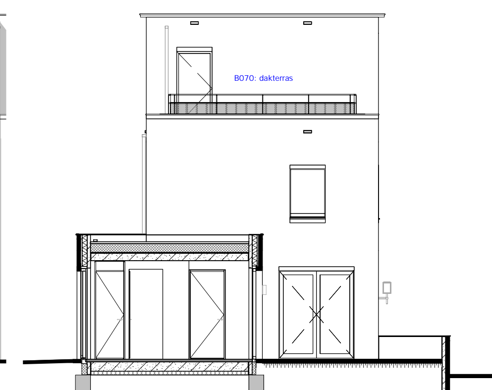
AANZICHT DAKTERRAS
