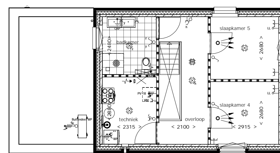
2e VERDIEPING
