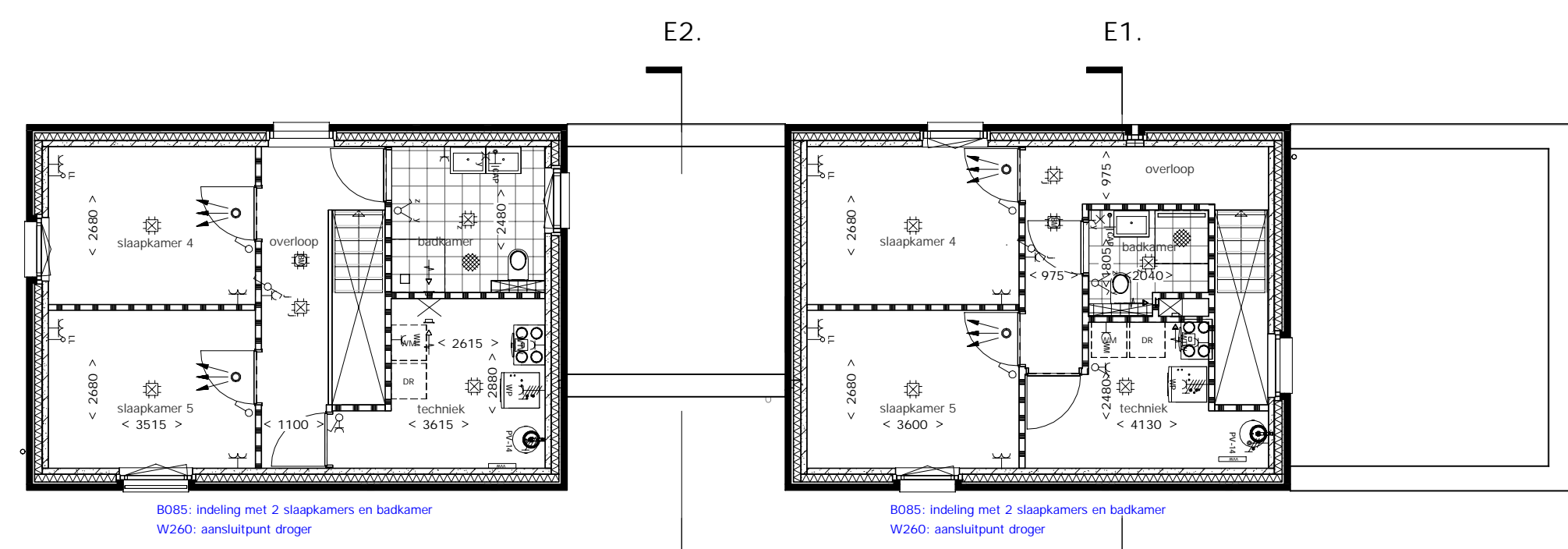
2e VERDIEPING
