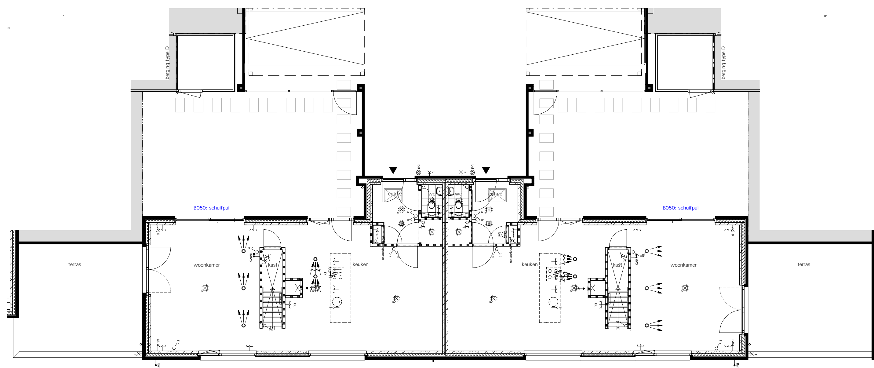
BEGANE GROND
