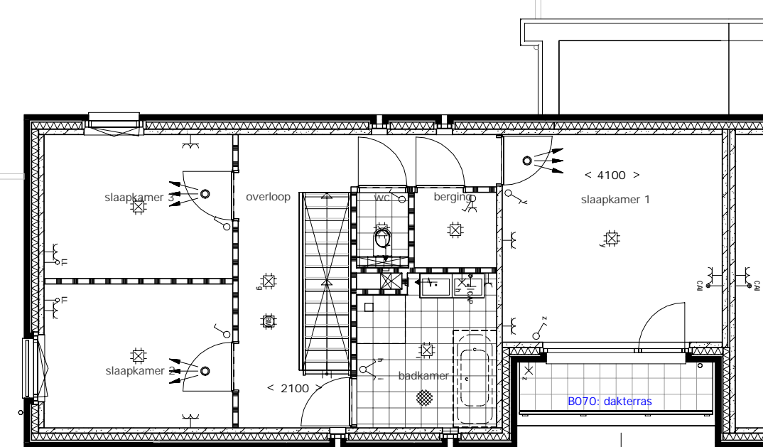
2e VERDIEPING
