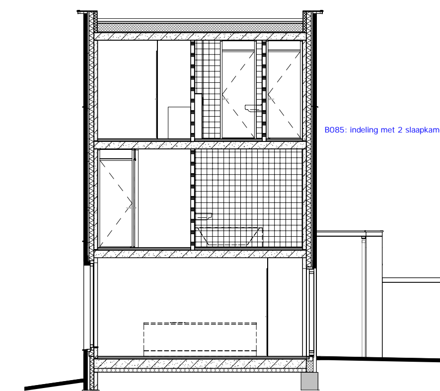
DOORSNEDE E1
