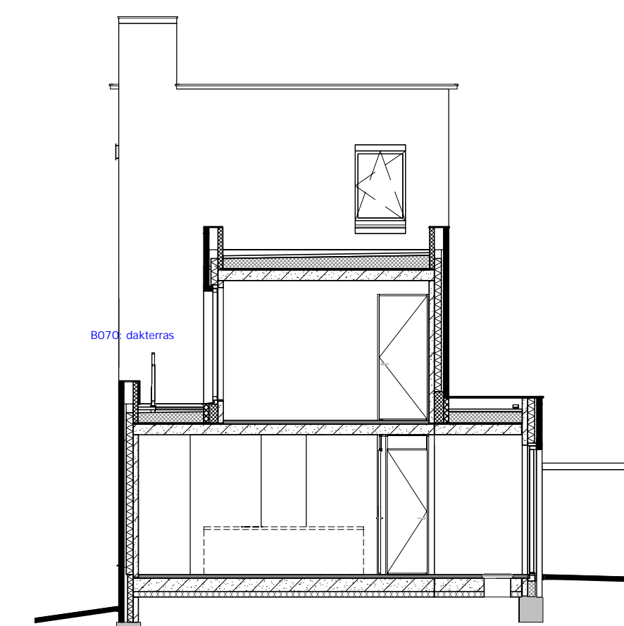
DOORSNEDE E2
