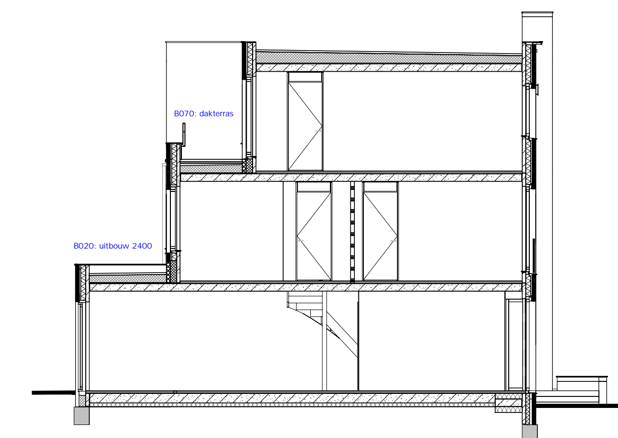
DOORSNEDE B2
