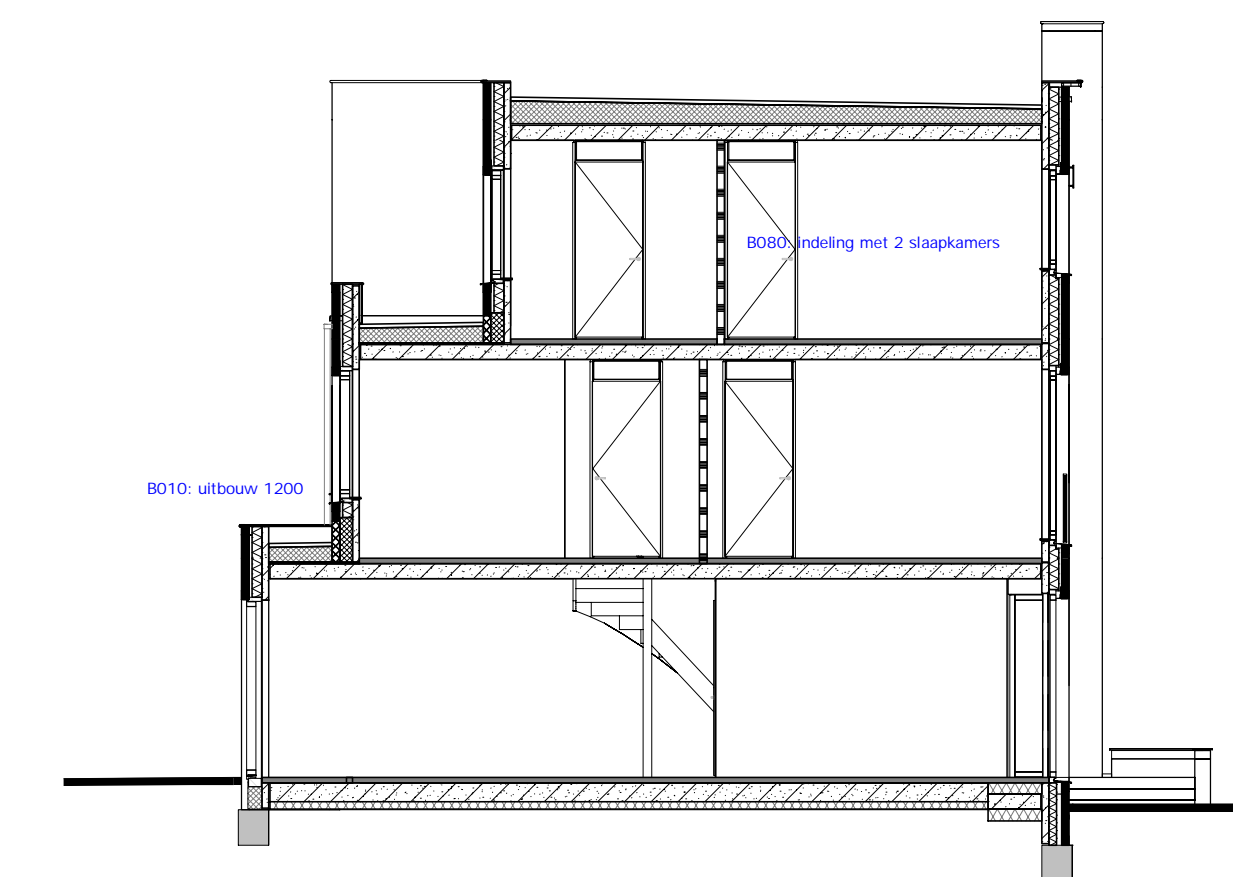
DOORSNEDE B1
