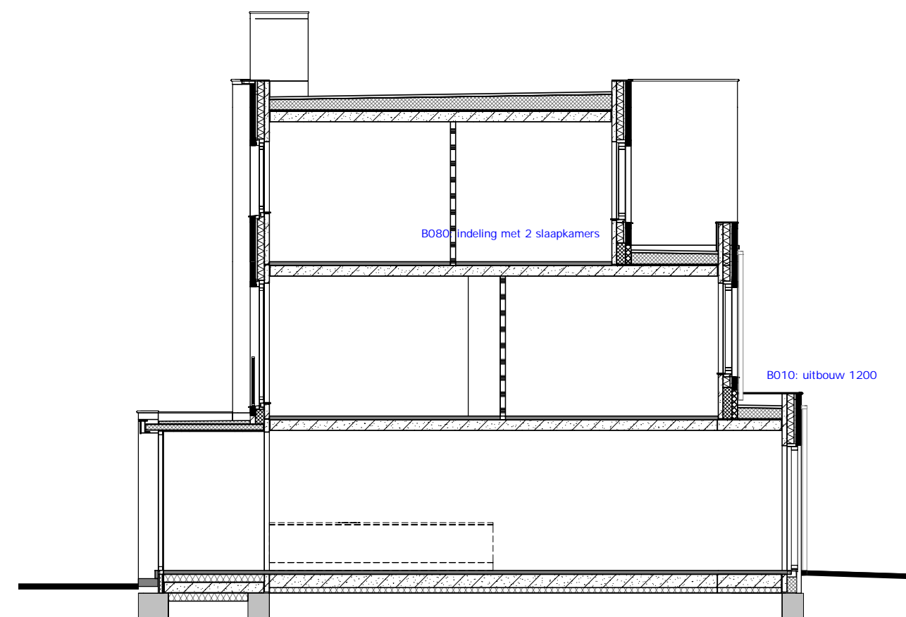
DOORSNEDE A1
