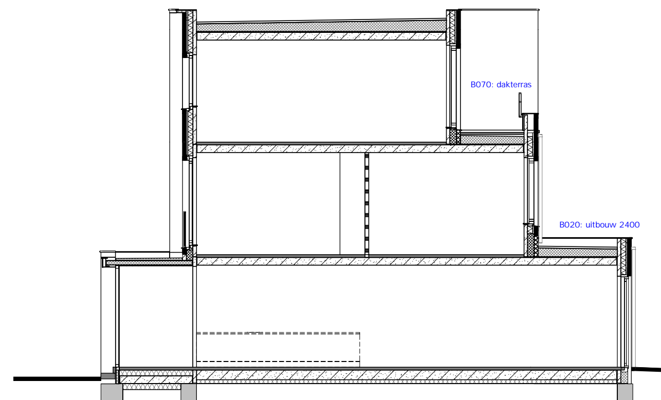
DOORSNEDE A2
