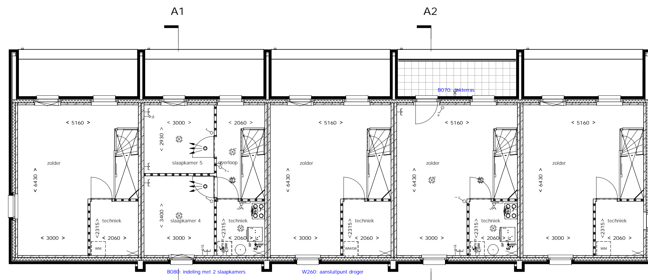
2e VERDIEPING
