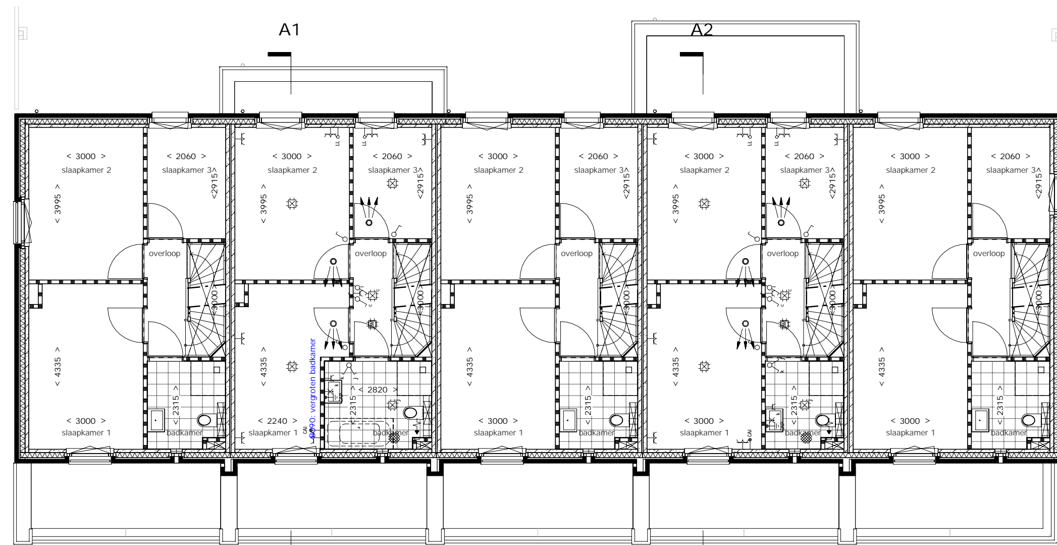
1e VERDIEPING
