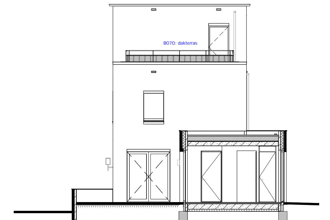
AANZICHT DAKTERRAS
