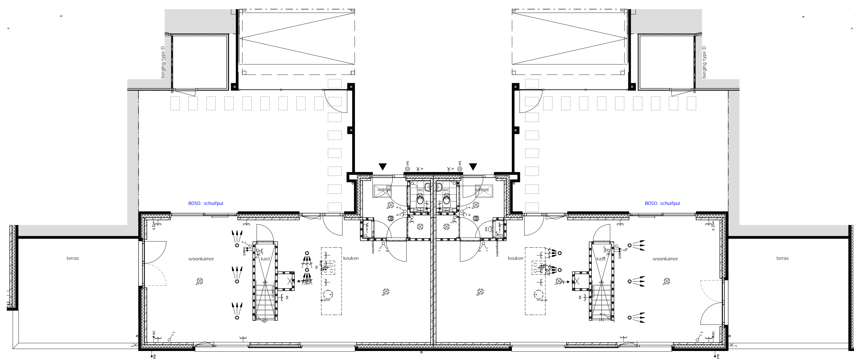
BEGANE GROND
