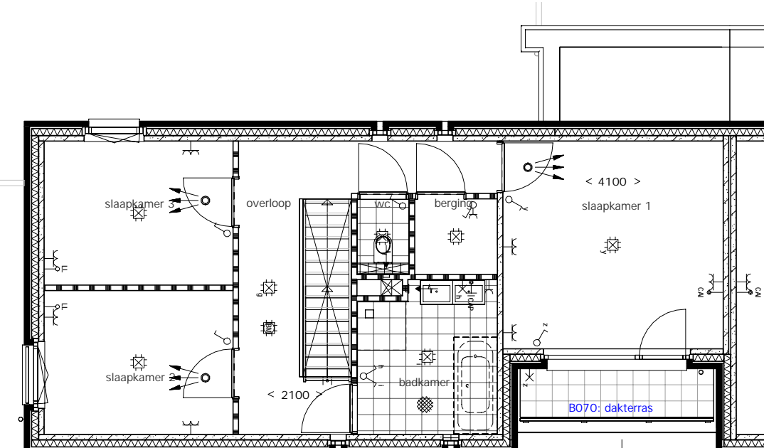
2e VERDIEPING
