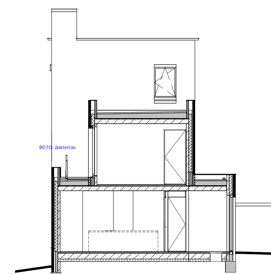
DOORSNEDE E2
