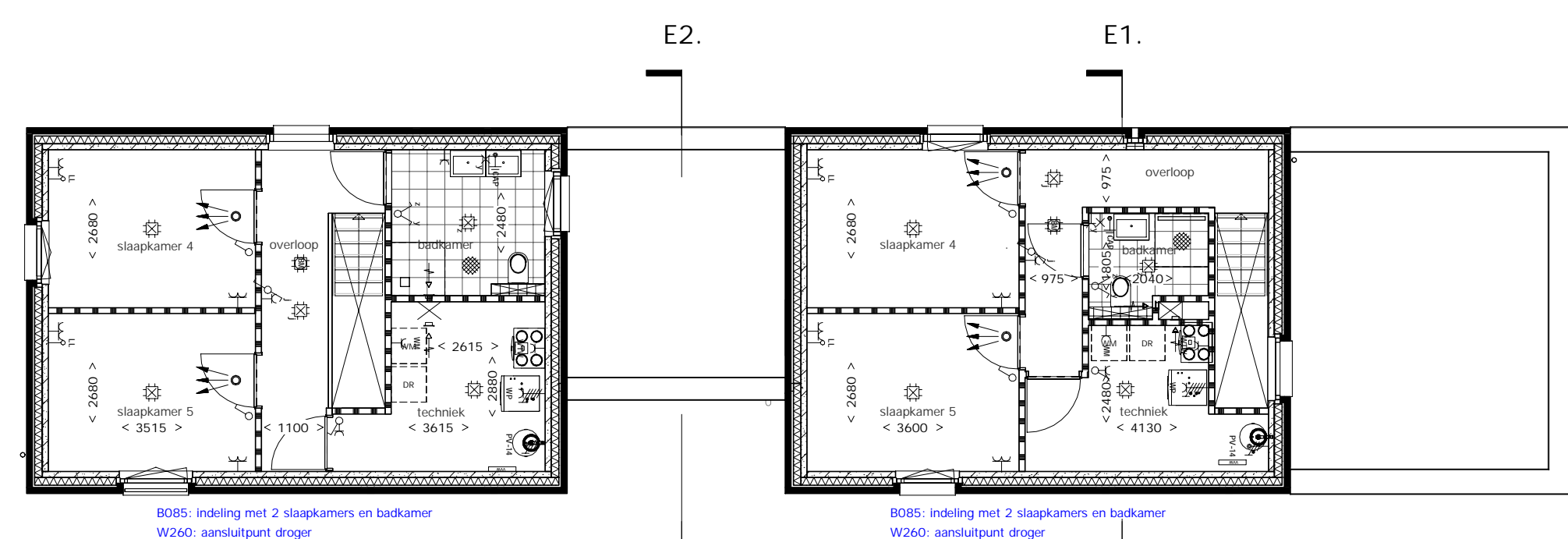
2e VERDIEPING
