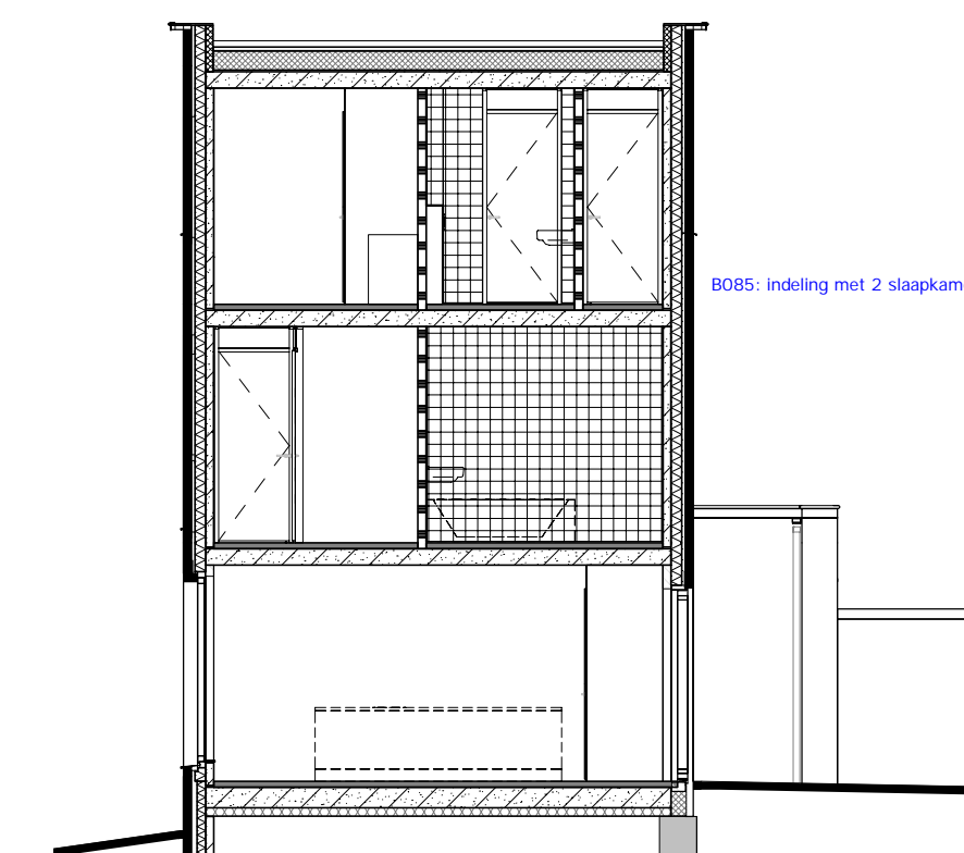
DOORSNEDE E1
